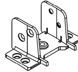
Orta Kayıt Bağlantı Takozu 34007-12140
