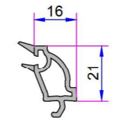
32mm Dekoratif Üçlü Cam Çıtası P.A.101.4202.600.0.HC
