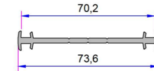
İnce Bağ Profili P.A.070.5001.600.0.00.19
