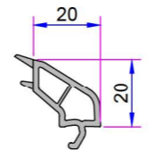
28mm Çift Cam Çıtası P.A.101.4100.600.0.HC
