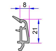
40mm Üçlü Cam Çıtası P.A.532.4400.600.0.HC
