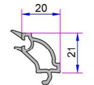
28mm Dekoratif Çift Cam Çıtası P.A.101.4102.600.0.HC
